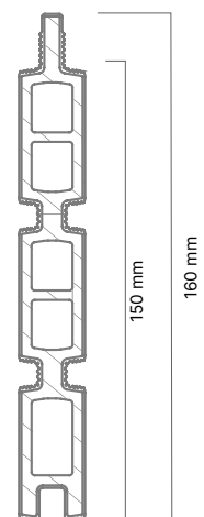
21 × 160 mm (DB 150 mm) L. 1780 mm
