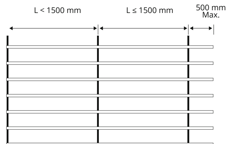
HORIZONTALE MONTAGE
