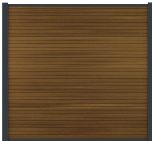
Boston scherm WPC-Modern (H183 x B176 cm), met 12x WPC profielen (21 x 160 mm), incl. Start- en eindprofiel aluminium
