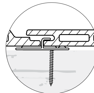
Fixation par clip
