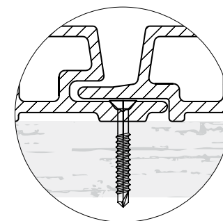
Fixation par vis
