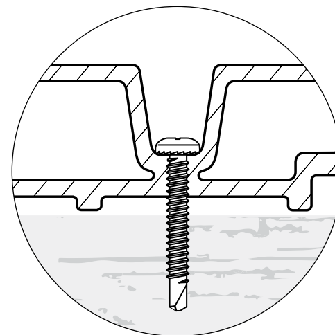
Fixation par vis
