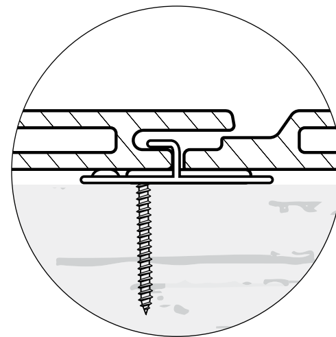
Fixation par clip
