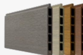
LAME PREMIUM EMBOITABLE 21 x 150 x 1780 mm Dark Grey Réf. 1232 | Ipé Réf. 1233 Teak Réf. 1234 | Light Grey Réf. 1235
